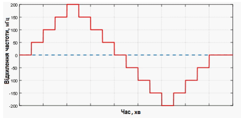
Рисунок 3. Малі сигнали відхилення частоти
