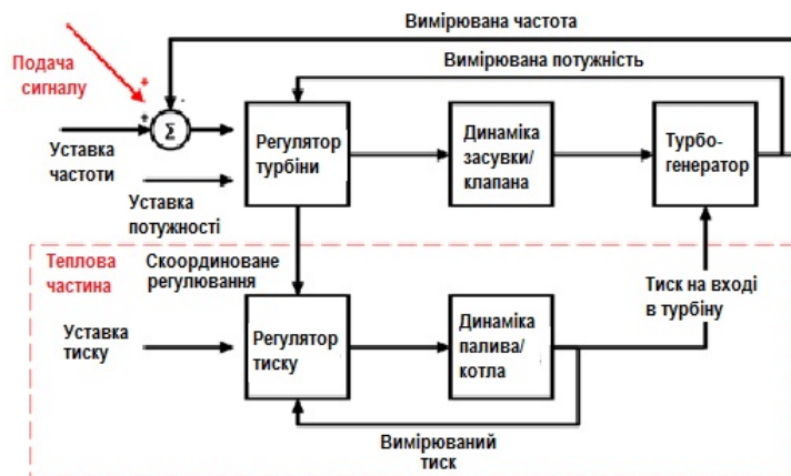
Рисунок 1. Приклад подачі сигналу регулятора
