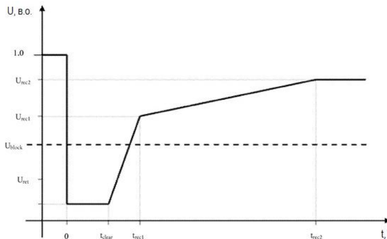
Крива залежності напруги від часу
